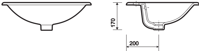
E100 550 1TH countertop basin
