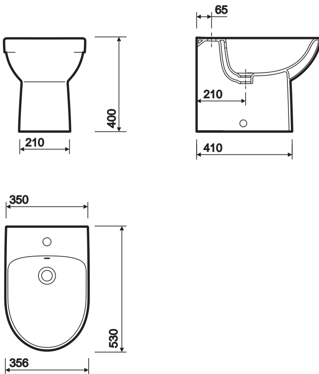
E100 floorstanding bidet
